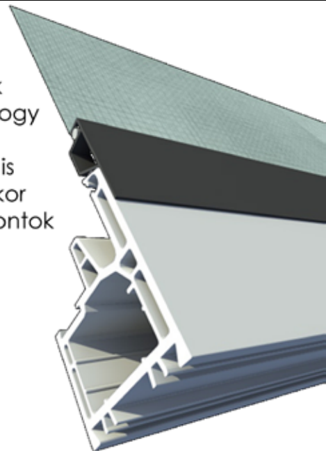
Rögzítő klipszek felszegecselése
