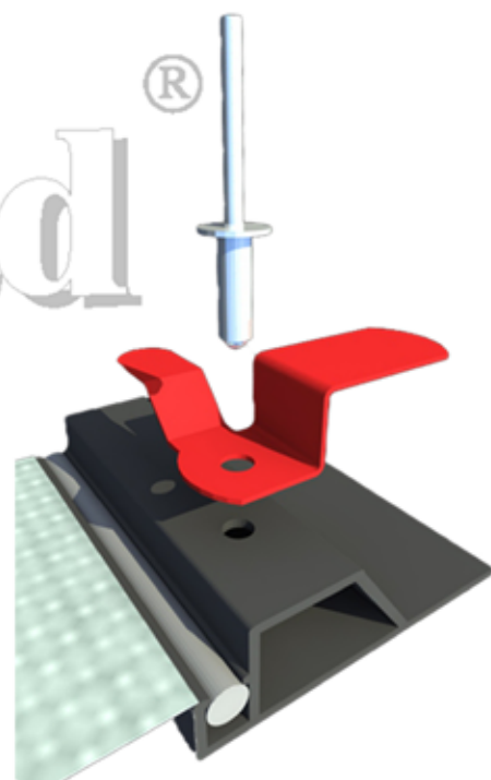
Rögzítő klipszek felszegecselése
